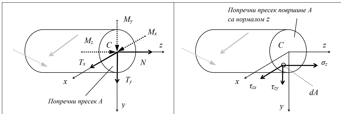
Слика 3.8. Равнотежа гредног елемента
