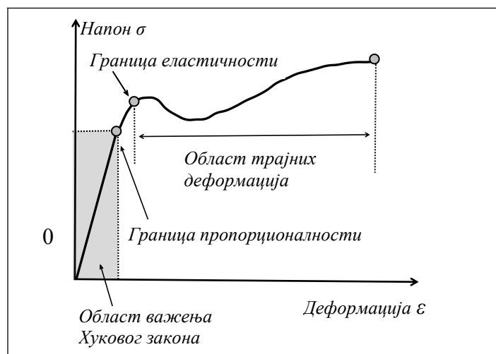
Слика 3.6. Веза нормалног напона и одговарајуће деформације
