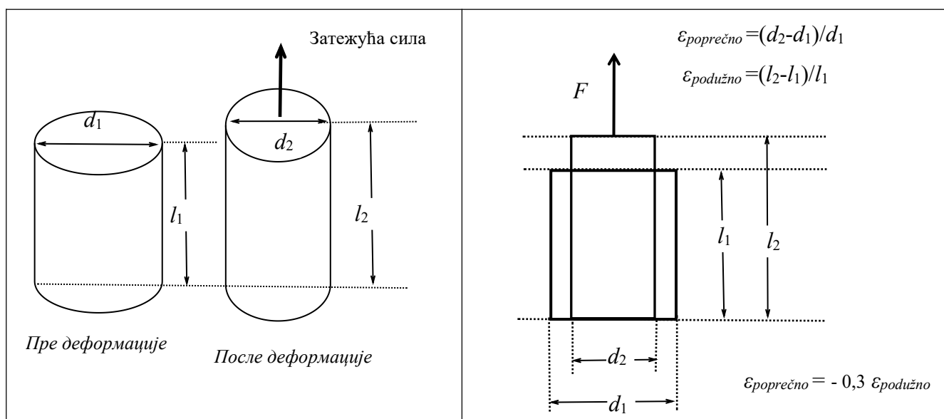
Слика 3.7. Подужна и попречна деформација
