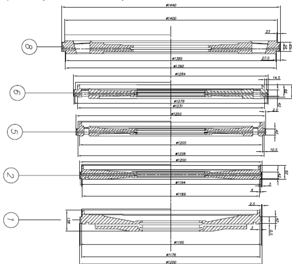
Slika 1: Oštećene dijafragme turboduvaljke
