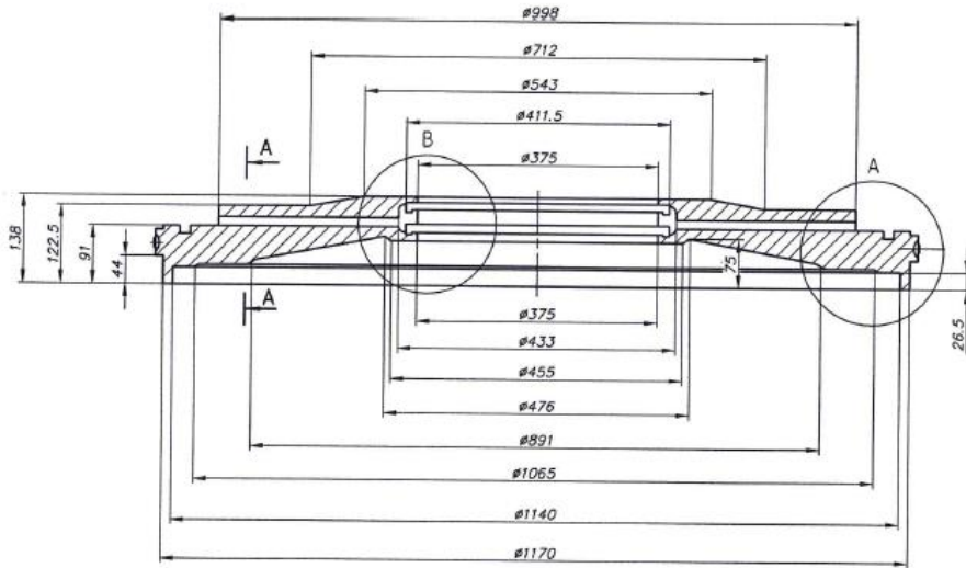
Pogled "A"
