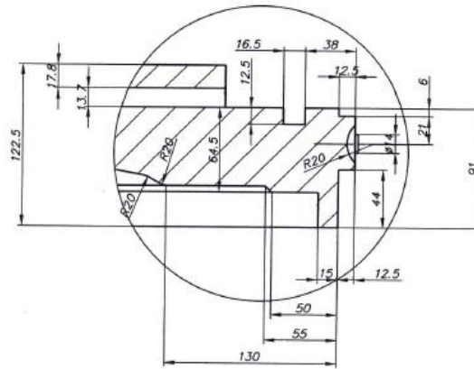
DETALJ A
