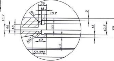
DETALJ A
