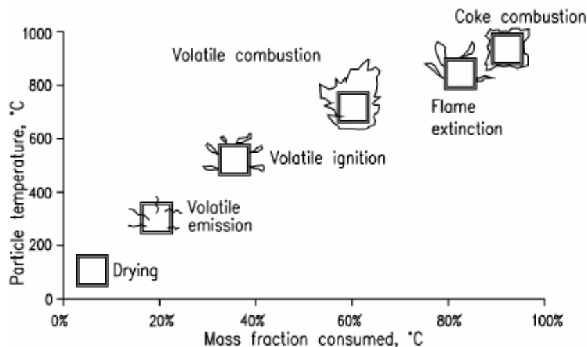
Слика 4.1: Фазе сагоревања биомасе [1]
