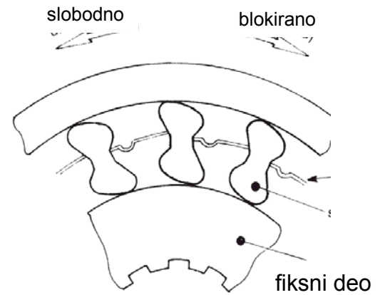
jednosmerna spojnica
