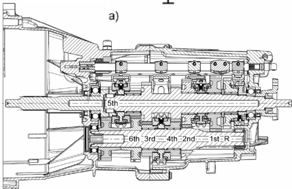
a) 6-stepeni manuelni menjač za benzinski motor
