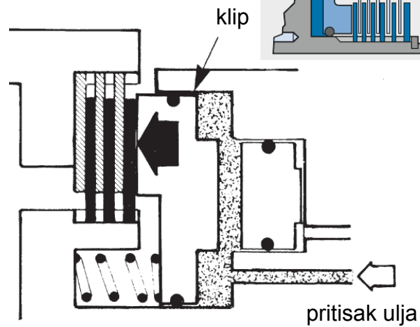
višelamelasta spojnica
