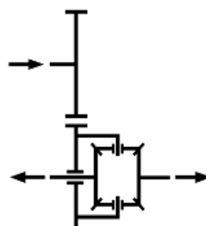
c) Razvod pogona (50:50) sa međuosnim diferencijalom
