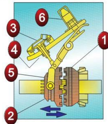
Potpuna blokada diferencijala - kandžasta spojnic
