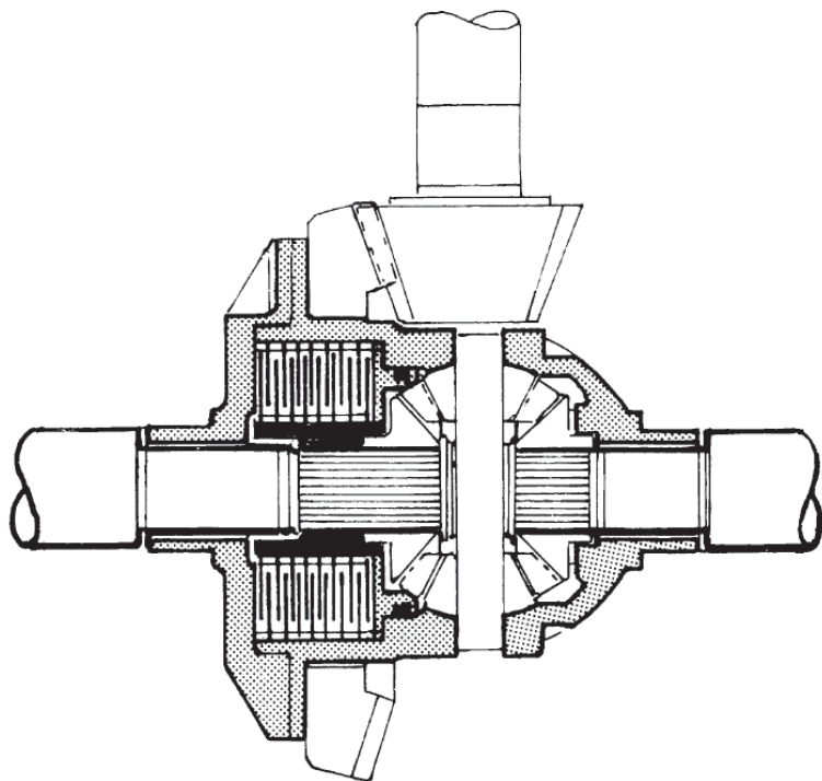
Delimična blokada diferencijala - visko-spojnic
