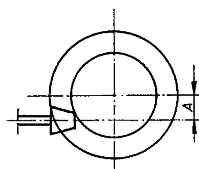
Konusno-tanjirasti par sa osama koje se mimolilaze (najčešće putnička vozila)
