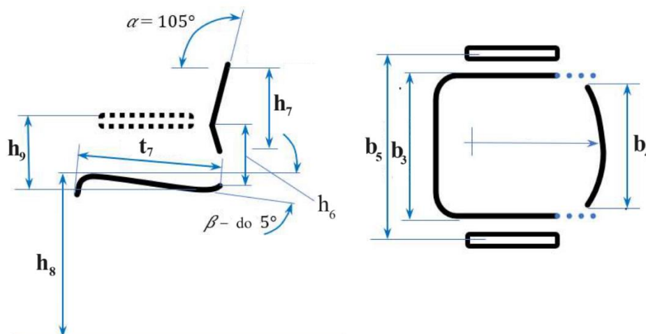
Слика 1. Приказ ергономске столице и њене димензије
