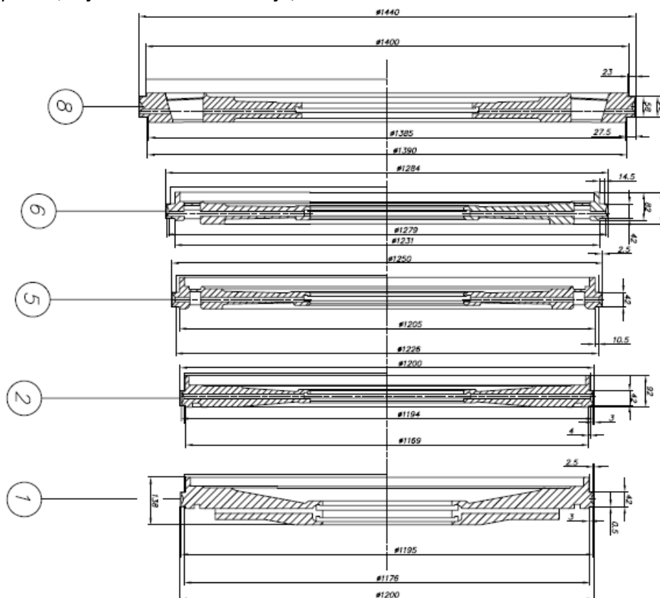
Slika 1: Oštećene dijafragme turboduvaljke
