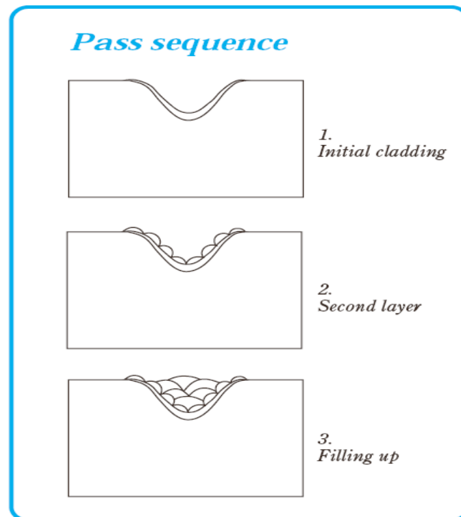
Slika 7: Popunjavanje žleba
