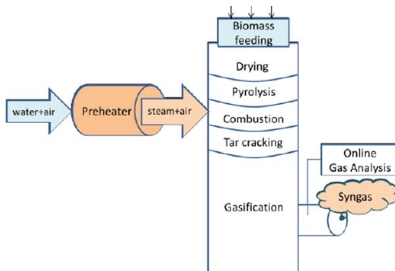
Слика 6.9: Схематски приказ процеса гасификације
