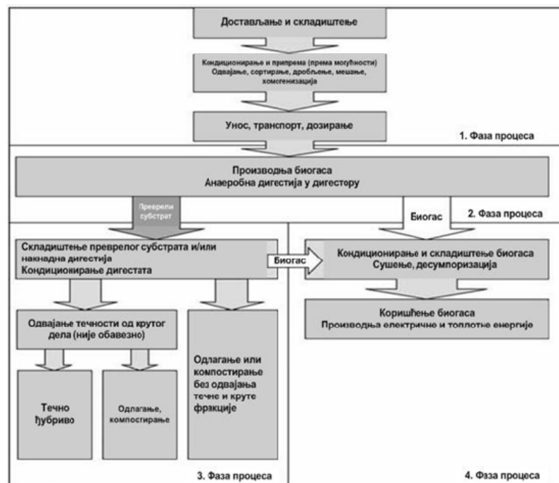
Слика 6.6. Фазе процеса производње биогаза од биомасе из пољопривреде
