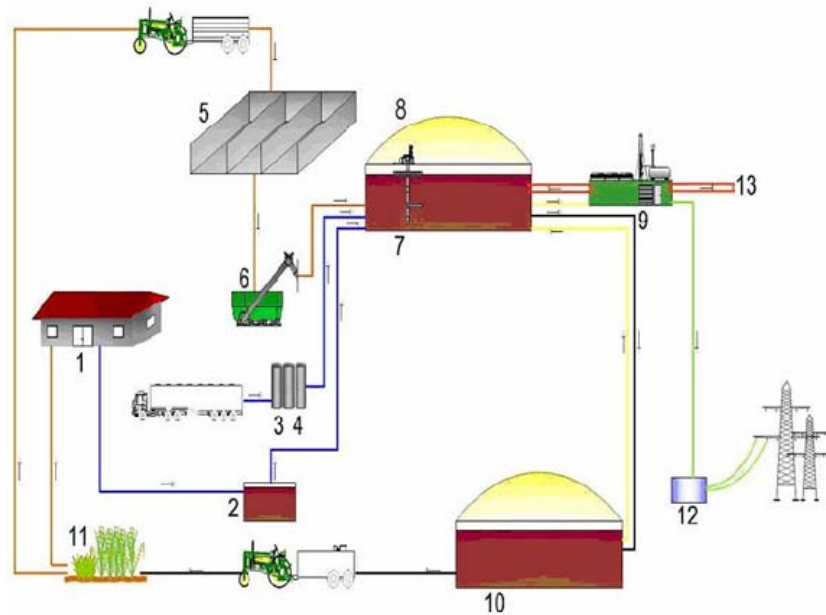
Слика 6.7. Фазе процеса производње биогаза у биогасном постројењу од биомасе из пољопривреде и стајњака на пољопривредном газдинству
