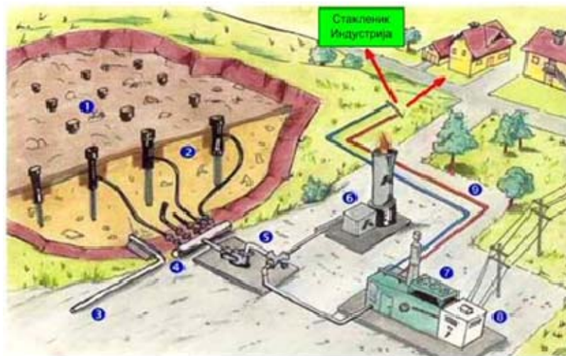
Слика 6.4. Технолошки процес производње биогаса на депонији
