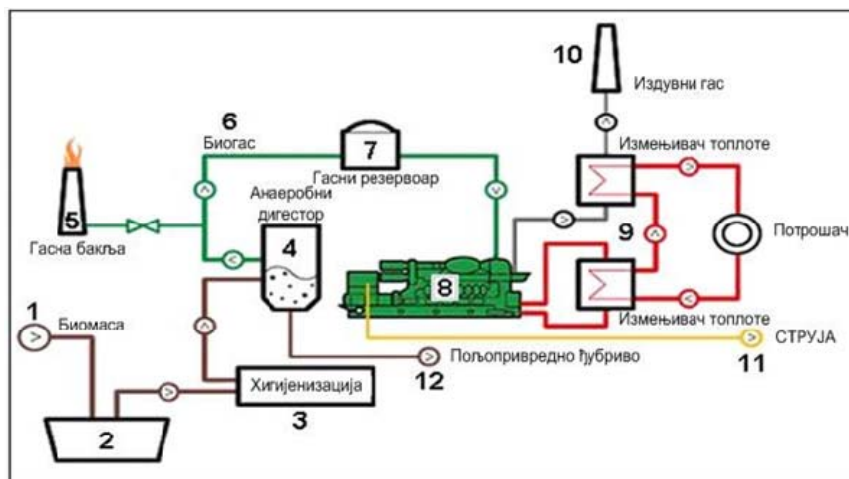
Слика 6.2. Технолошки процес производње биогаза
