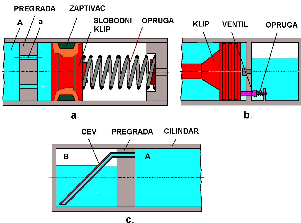
Sl 6. Kompenzatori tečnosti
