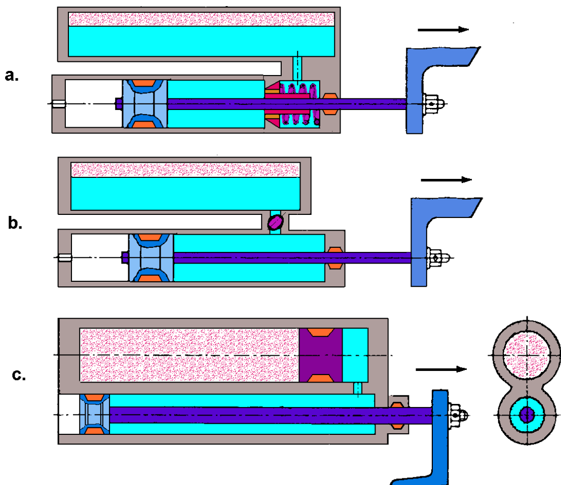
SI 9. Hidropneumatski povratnici
