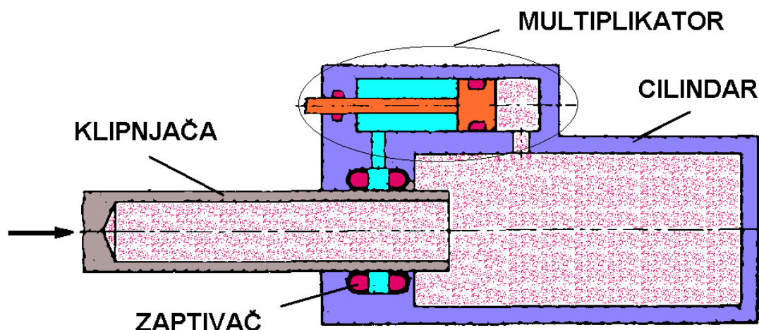
SI 8. Pneumatski povratnik
