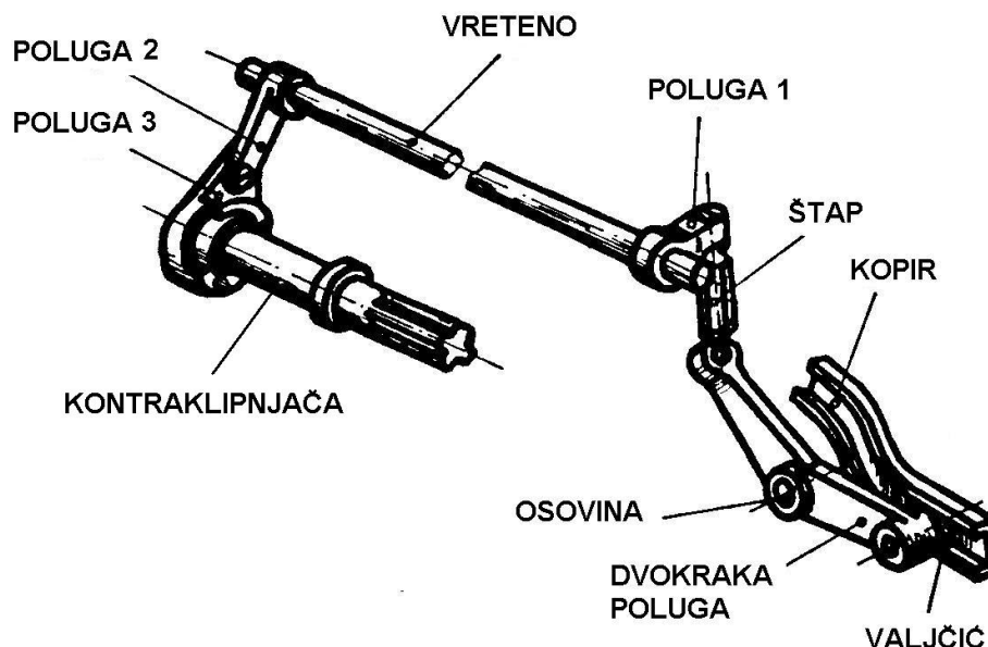
Sl 4. Mehaniizam za promenu dužine trzanja
