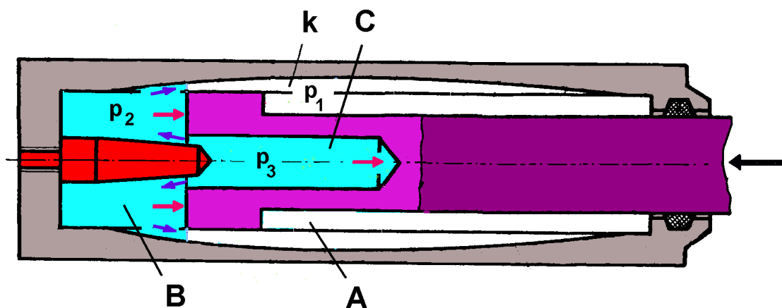
SI 2. Funkcija hidraulične kočnice sa slike 1 pri vraćanju
