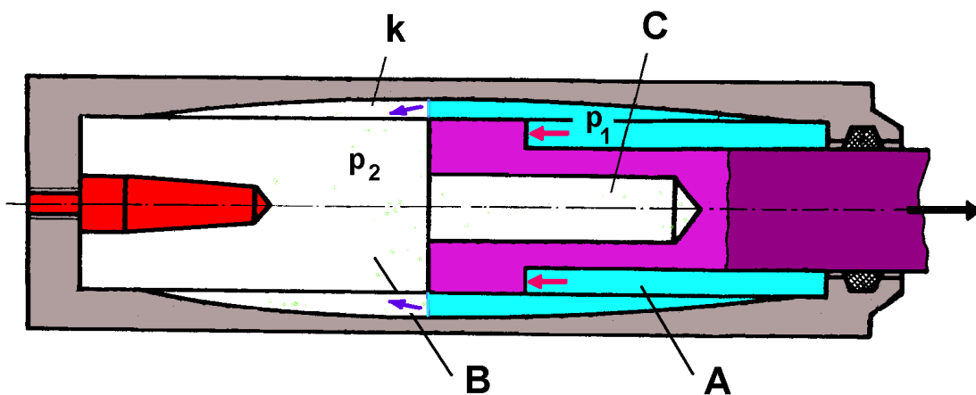
SI 2. Funkcija hidraulične kočnice sa slike 1 pri trzanju
