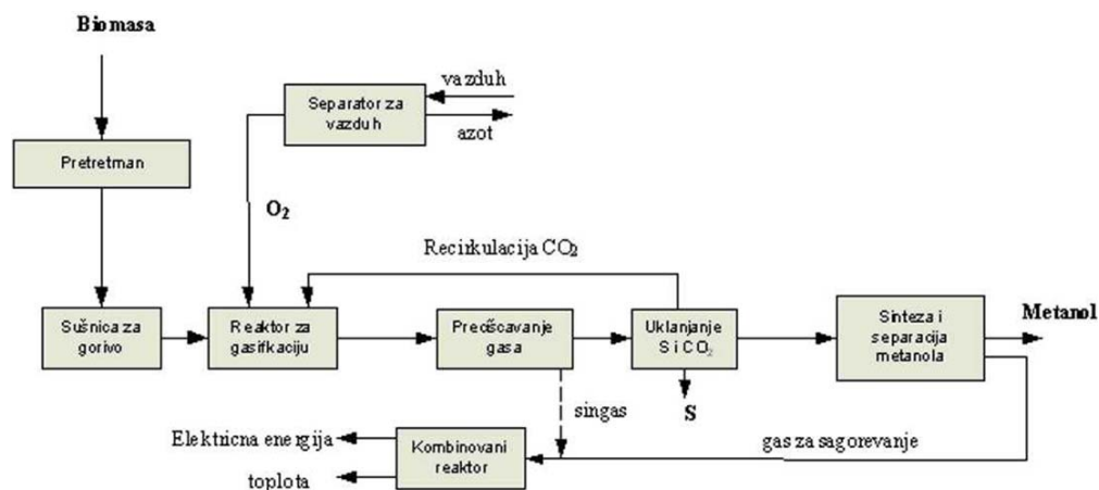
Слика 4: Технолошки процес производње метанола из биомасе
