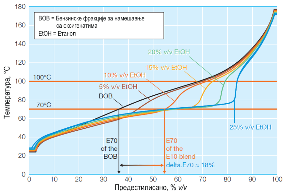
Слика 6: Утицај додавања етанола моторном бензину на криву дестилације мешавине
