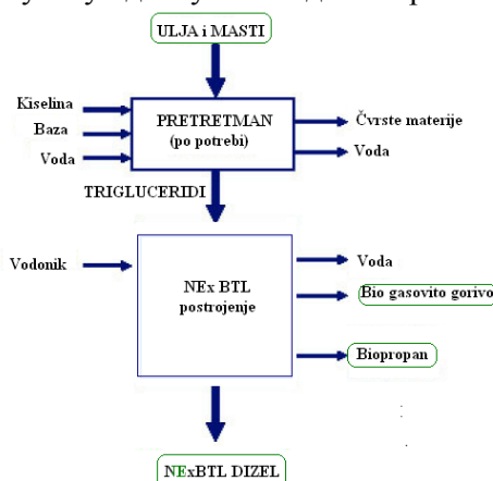
Слика 9. Блок дијаграм процеса добијања NExBTL дизела
