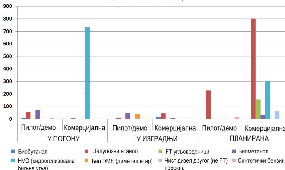
Слика 3: Напредне технологије за производњу биогорива
