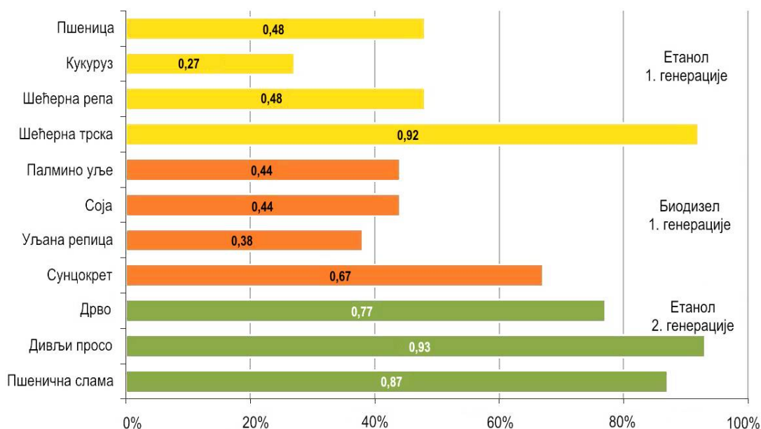
Слика 11: Процене просечних уштеда у емисији GHG гасова које се могу постићи применом биогорива
