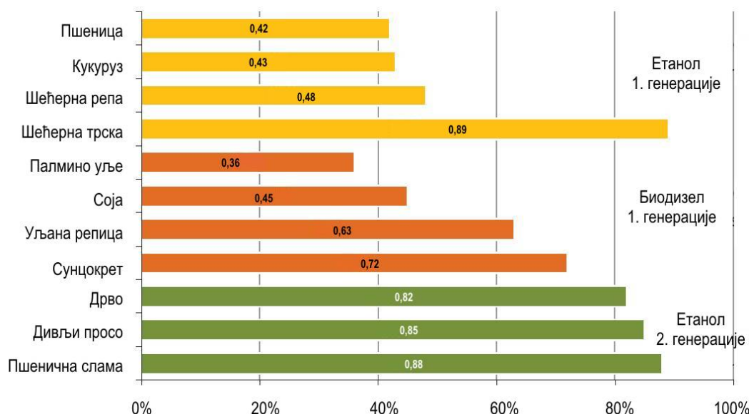
Слика 10: Смањење коришћења енергије фосилних горива %укупне уштеде енергије фосилних горива у односу на референтне системе на фосилно гориво за различите сировине и технологије производње биогорива
