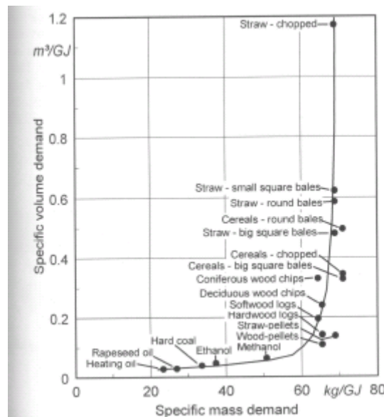
Слика 4.1: Специфична маса/запремина различитих врста биомасе (садржај воде 15 % m/m)
