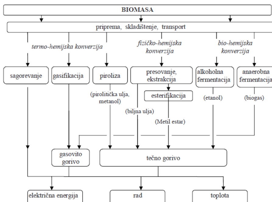
Слика 4.3: Основне технологије конверзије биомасе
