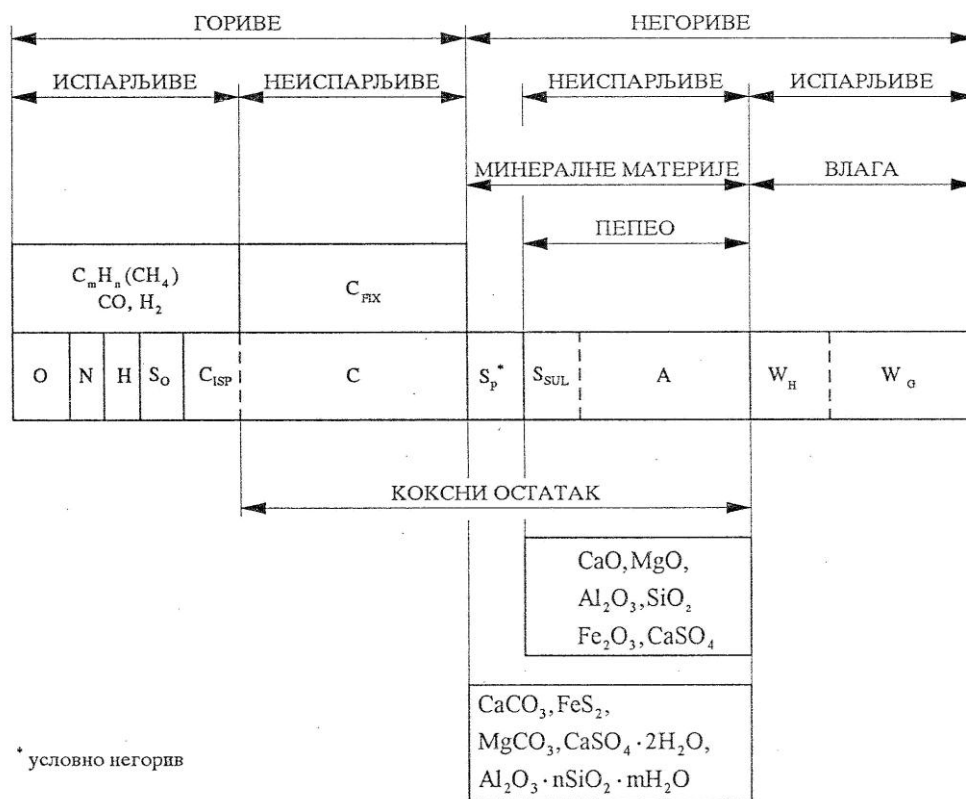
Слика 4.8. Техничка анализа чврстих горива
