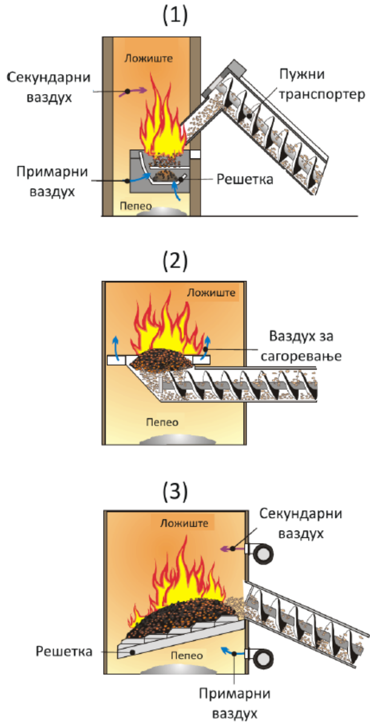
Слика 8.8. Начин довода горива у уређајима за сагоревање пелета
